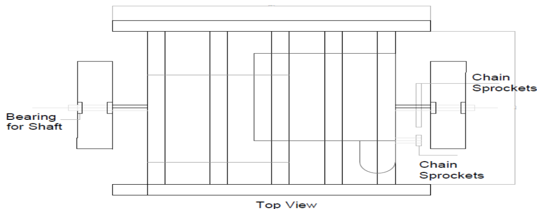
Fig. 12 Base/Chassis
